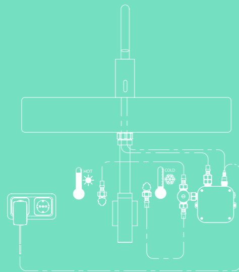
EN Type 2: Indirect temperature control via under-counter control box. ES Tipo funcional 2 con regulación de temperatura indirecta mediante una unidad de control bajo encimera.
