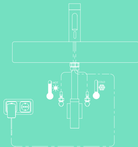
EN Type 1: Direct temperature control at faucet. ES Tipo funcional 1 con regulación de temperatura directa mediante maneta giratoria.
